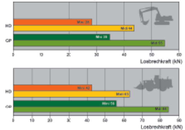
Losbrechkraft Diagramm
